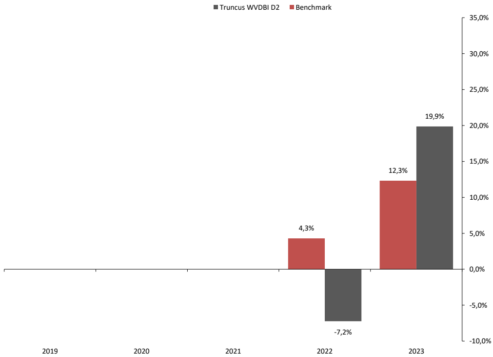
staafdiagram met jaarlijks rendement klasse D2
