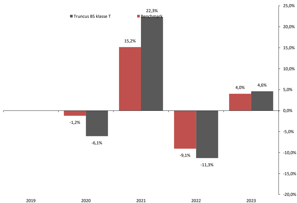
Klasse T: staafdiagram met jaarlijks rendement
