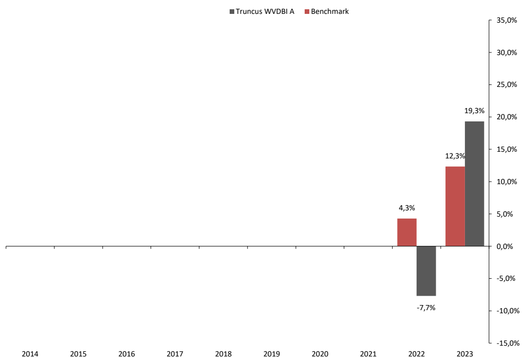
staafdiagram met jaarlijks rendement klasse A
