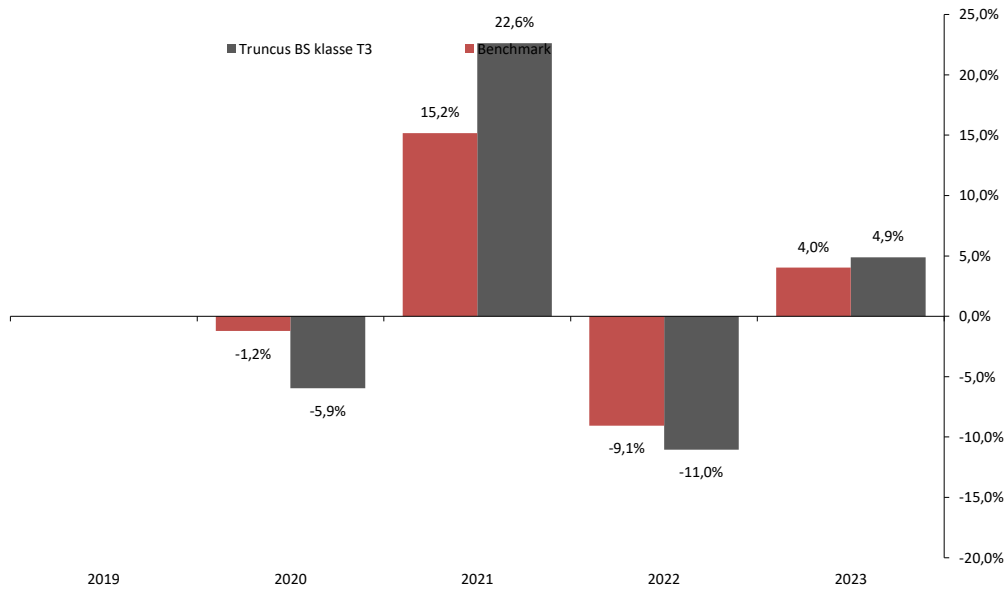
Klasse T3: staafdiagram met jaarlijks rendement
