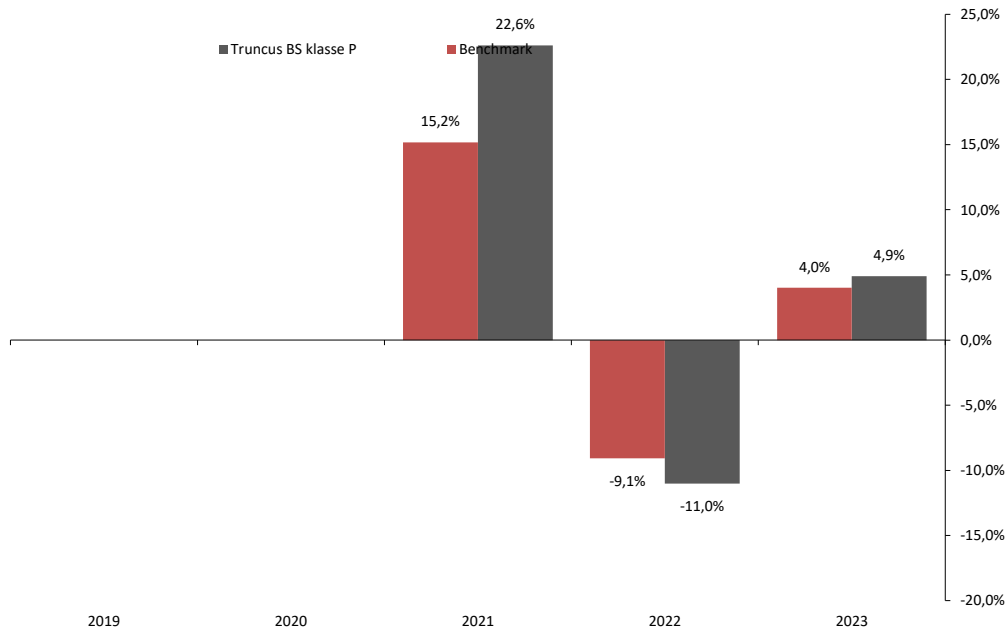
Klasse P: staafdiagram met jaarlijks rendement
