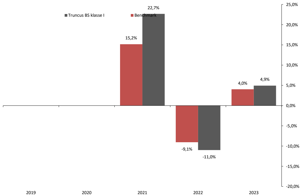
Klasse I: staafdiagram met jaarlijks rendement
